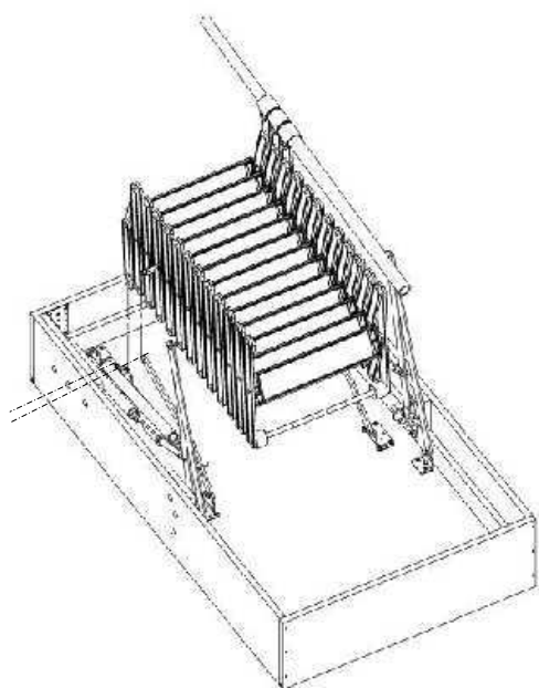
Scherentreppe M
