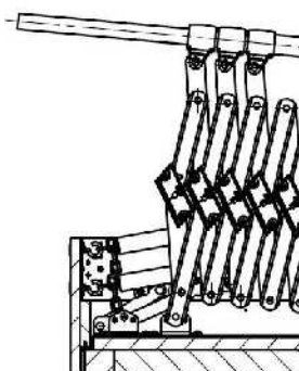
Scherentrepppe M
